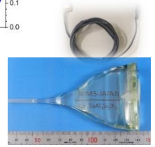
温度変化がなく車載規格を満たすBSO
