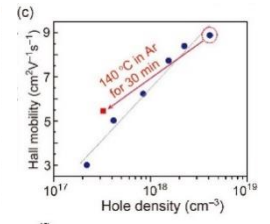
液相合成可能なa-Cu-Sn-Iが示す高いホール移動度 (9 cm²V⁻¹s⁻¹)
