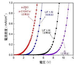
Zn-Si-Oを電子輸送層に用いる高効率OLEDのI-V特性
