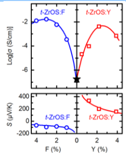
両極性伝導を示すZrOS
