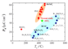
高T C で大きな自発分極を示すHfO 2 :Y
